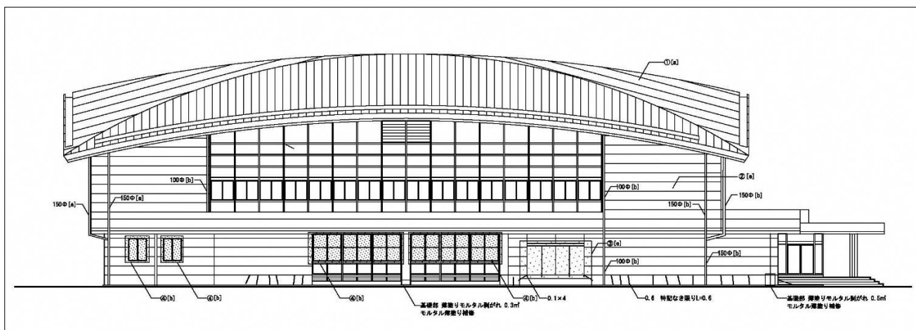
【立面図(北側)】
