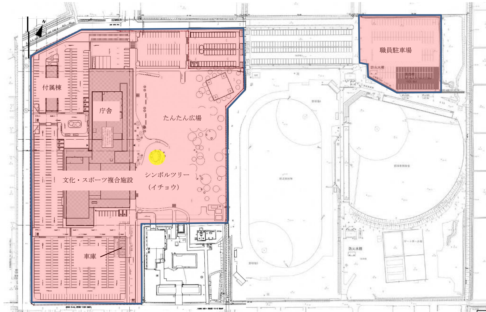
配置図
