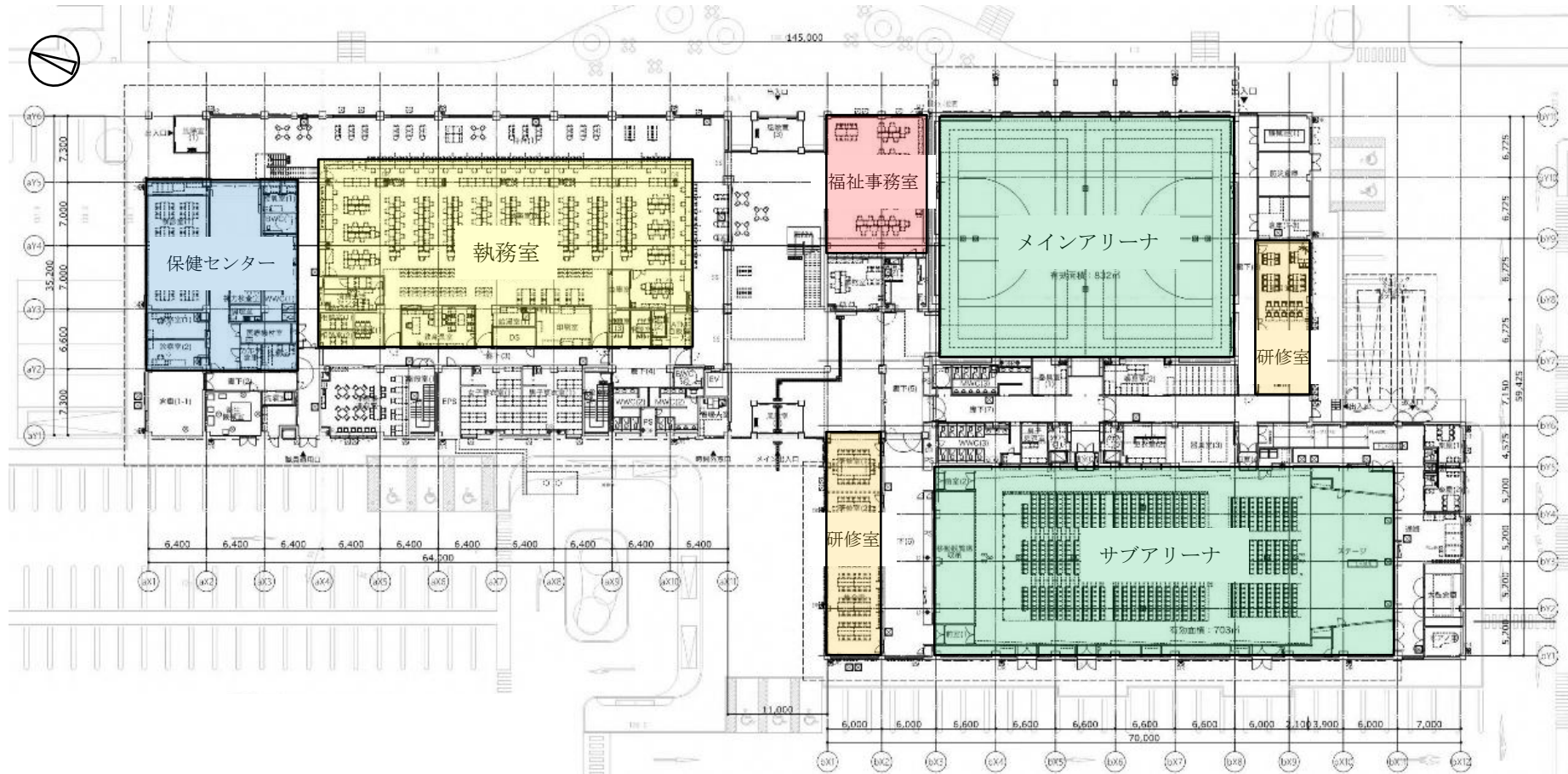
1 階平面図
